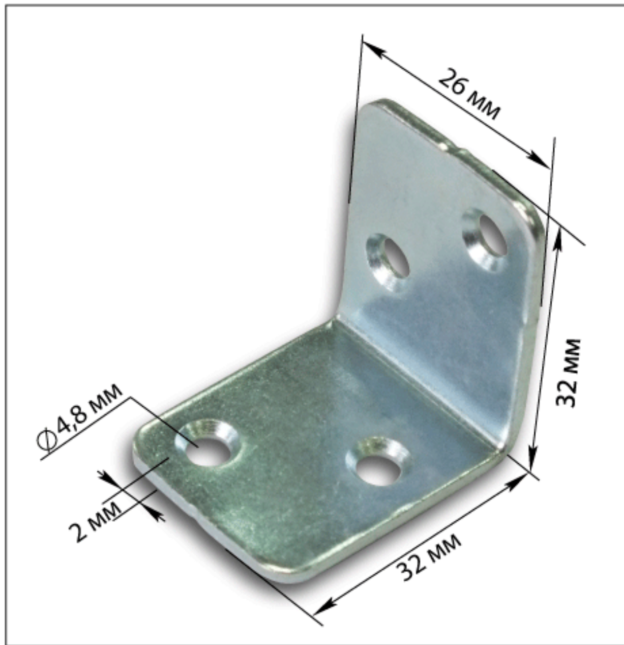
Уголок крепежный 32 x 32 x 26 мм, с 4-мя отв. d 4,8 мм, оц.ст. 2мм
