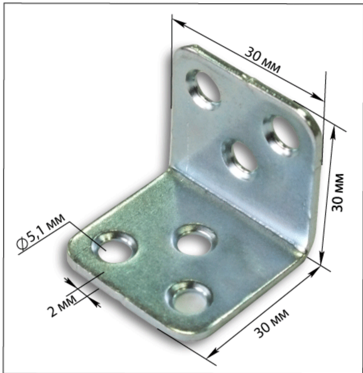
Уголок крепежный 30 x 30 x 30 мм, с 6-ю отв. d 5,1 мм, оц.ст. 2,0 мм
