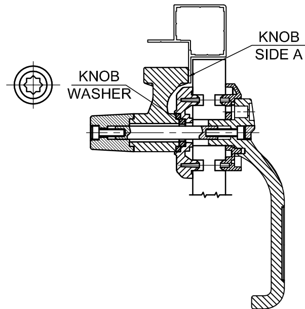
PANNELLO SINGOLA PIEGA PROFILO STANDARD
