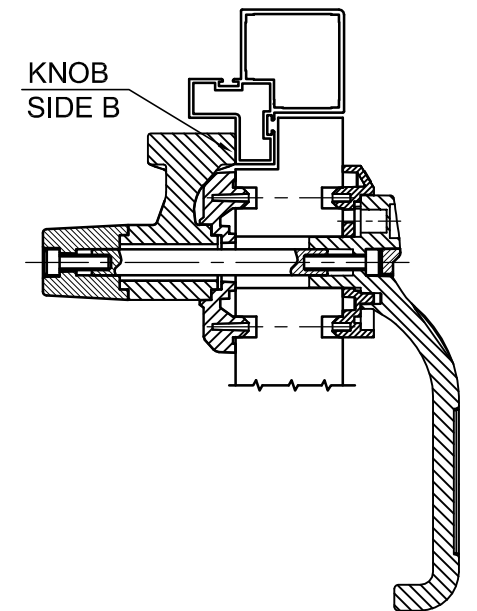
PANNELLO DOPPIA PIEGA PROFILO DOPPIA CAMERA
