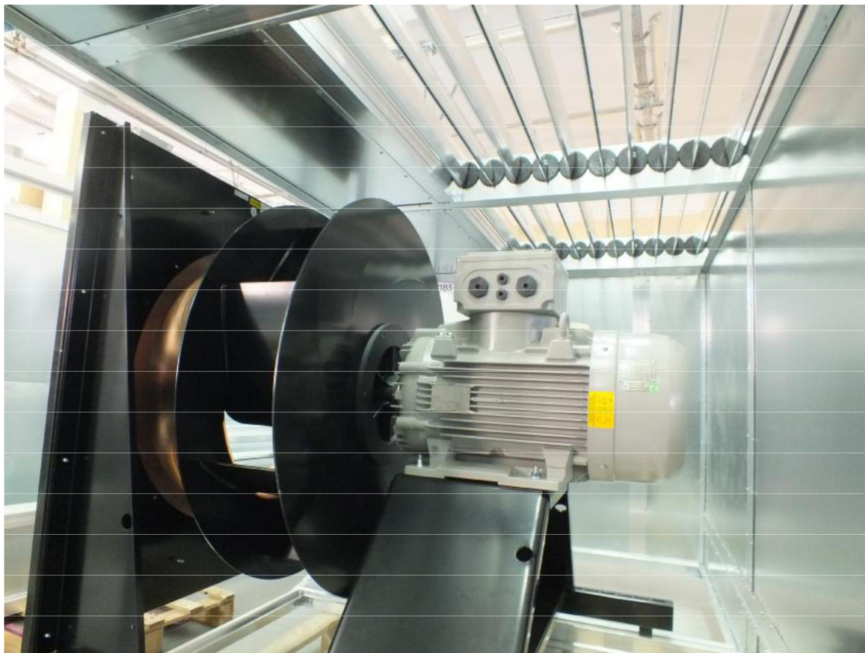
Установки Миникон 3600/7 в производстве: часть вытяжной вентиляторной секции с заслонкой
