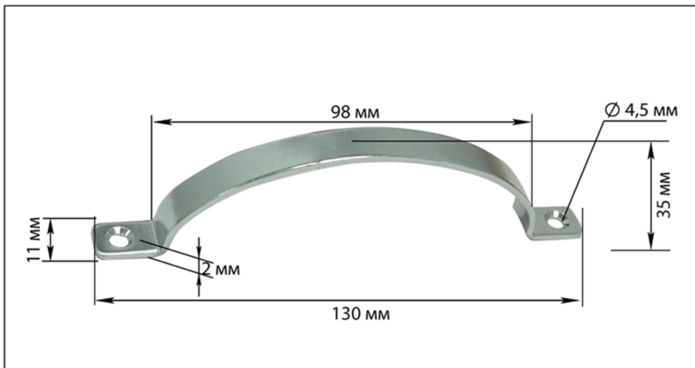
Ручка скоба 35 x 98 с отв. d 4,5 мм , оц.ст. 2 мм
