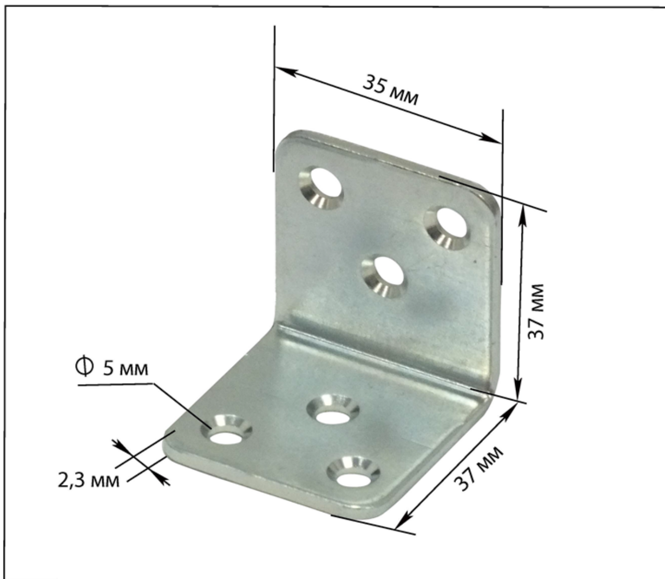
Уголок крепежный 37 x 37 x 35 мм, с 6-ю отв. d 5 мм, оц.ст. 2,3 мм
